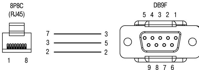
Рисунок Б.3 – Кабель КС6 для консольного доступа к Linux
