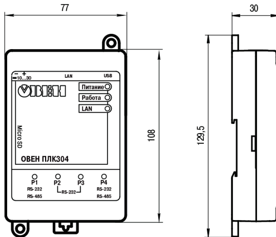
Рисунок А.1 – Габаритные размеры ПЛК304
