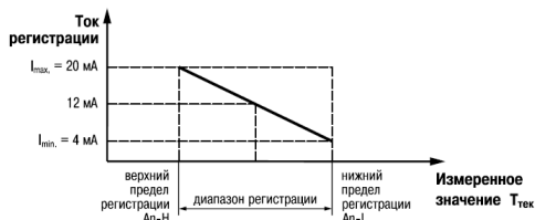
Рисунок 7.7 – A_{п-L} > A_{п-H}
