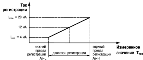
Рисунок 7.6 – A_{п-L} < A_{п-H}
