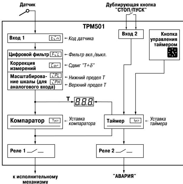
Рисунок 6.1 – Функциональная схема прибора
