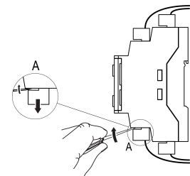
Рисунок 3 – Відкриття знімних частин клем
