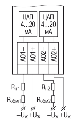
Рисунок 9 – Підключення навантаження до ВЕ типу «I»
