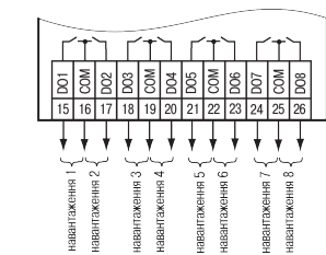
Рисунок 8 – Підключення навантаження до ВЕ типу «P»
