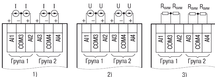
Рисунок 7 – Підключення: 1) активних датчиків з виходом типу «Струм 4...20 mA», 2) активних датчиків з виходом типу «Напруга 0...10 mA», 3) датчиків опору з діапазоном 0...4000 Ом
