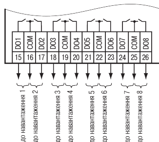
Рисунок 8 – Підключення навантаження до ВЕ типу «P»
