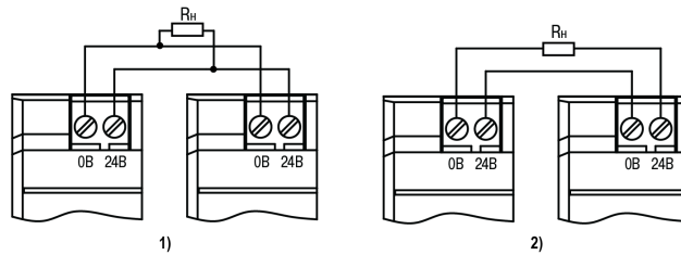
Рисунок 3 - Схема параллельного (1) и последовательного (2) подключения нескольких приборов
