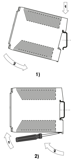
Рисунок 2 - Монтаж (1) и демонтаж (2) прибора
