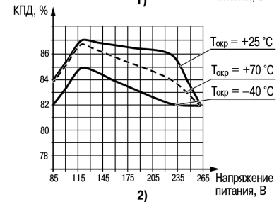
Рисунок 7 - График зависимости КПД от напряжения питания и температуры окружающей среды: (1) БП30А-12С, (2) БП30А-24С
