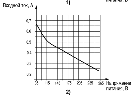
Рисунок 6 - График зависимости входного тока от напряжения питания: (1) БП30А-12С, (2) БП30А-24С
