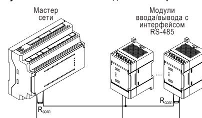
Рисунок 6 – Типовая схема подключения в режиме Master
