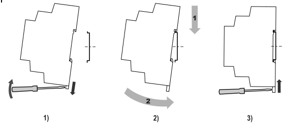
Рисунок 1 – Монтаж прибора
