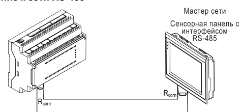
Рисунок 5 – Типовая схема подключения в режиме Slave
