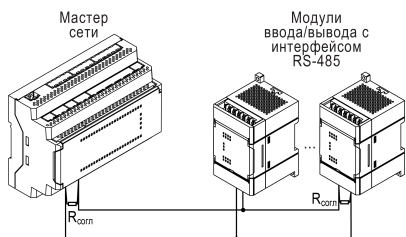
Рисунок 11 – Типовая схема подключения в режиме Master
