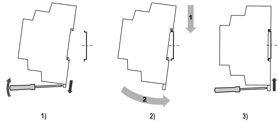
Рисунок 1 – Монтаж прибора
