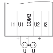
Рисунок 6 – Подключение датчиков с выходом в виде напряжения
