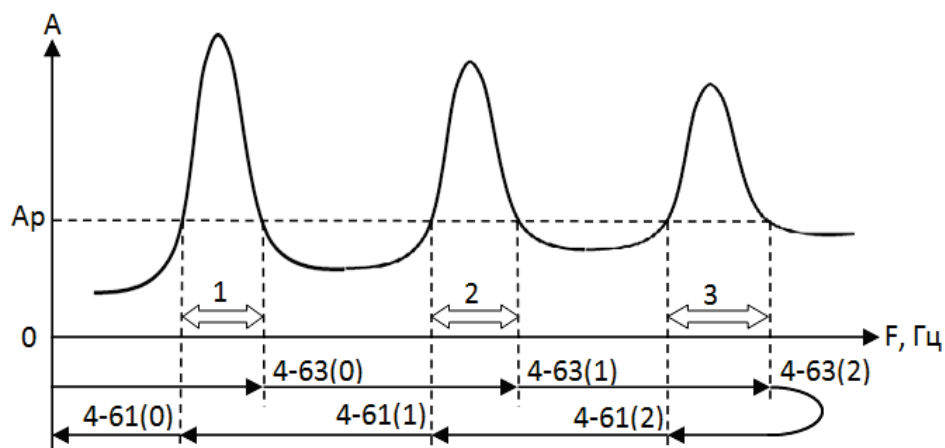
Рисунок 4.6 – Амплитуда вибрации (A) от частоты вращения АД при резонансе
