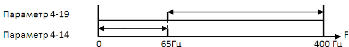
Рисунок 4.5 - Диаграмма алгоритма ввода значений частот
