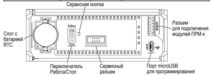
Рисунок 9 – Лицевая панель под крышкой
