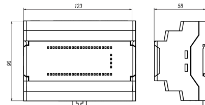
Рисунок 2 – Габаритные размеры прибора
