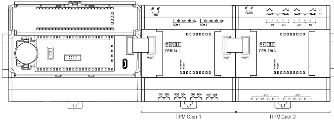
Рисунок 7 – Расположение модулей расширения на шине
