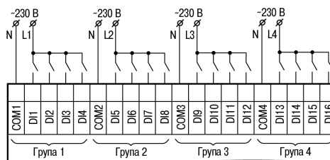
Рисунок 3 – Підключення до дискретних входів датчиків типу «сухий контакт» для сигналів 230 В
