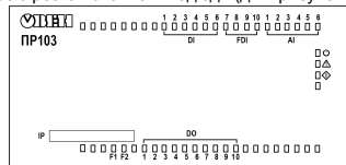
Рисунок 8 – Приклад лицьової панелі пристрою
