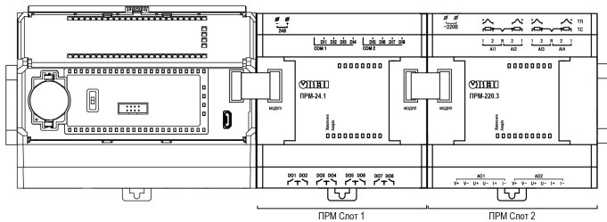
Рисунок 7 – Розташування модулів розширення на шині
