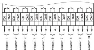
Рисунок 4 – Схема підключення навантажень до ВЕ типу «Р»
