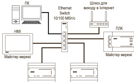
Рисунок 6 – Підключення за схемою «зірка»
