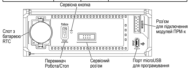
Рисунок 9 – Лицьова панель під кришкою
