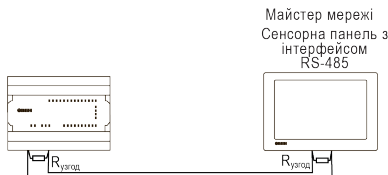
Рисунок 5 – Типова схема підключення у режимі Slave
