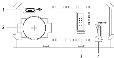
Рисунок 9 – Лицьова панель під кришкою
