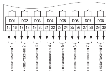
Рисунок 5 – Схема підключення навантаження до БЕ типу «Р»
