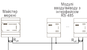
Рисунок 7 – Типова схема підключення для PR100 у режимі Master
