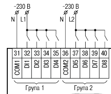
Рисунок 4 – Підключення дискретних датчиків із живленням 230 В
