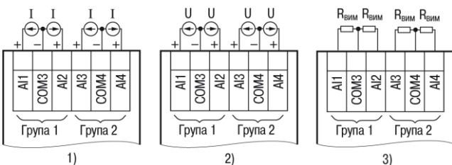
Рисунок 6 – Підключення: 1) активних датчиків з виходом типу «Струм 0...20 мА», 2) активних датчиків з виходом типу «Напряга 0...10 мА», 3) датчиків опору з діапазоном 0...4000 Ом
