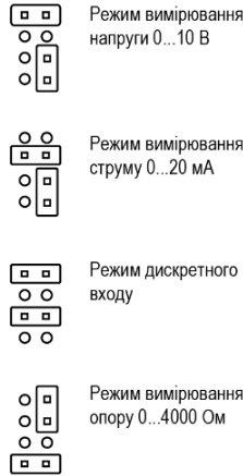
Рисунок 3 – Схема налаштування A11...A14
